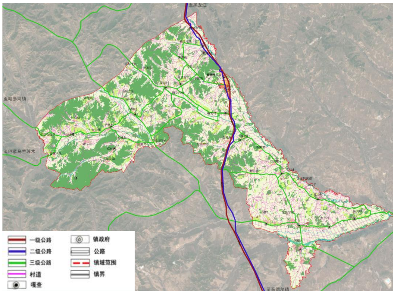
镇域交通规划图
